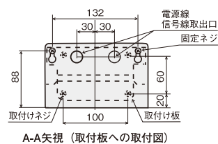
A-A矢視 (取付板への取付図)
