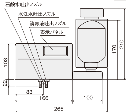
A-A矢視(取付板への取付図)
